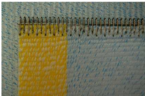
Filtrationsgewebe mit Randabdichtung
