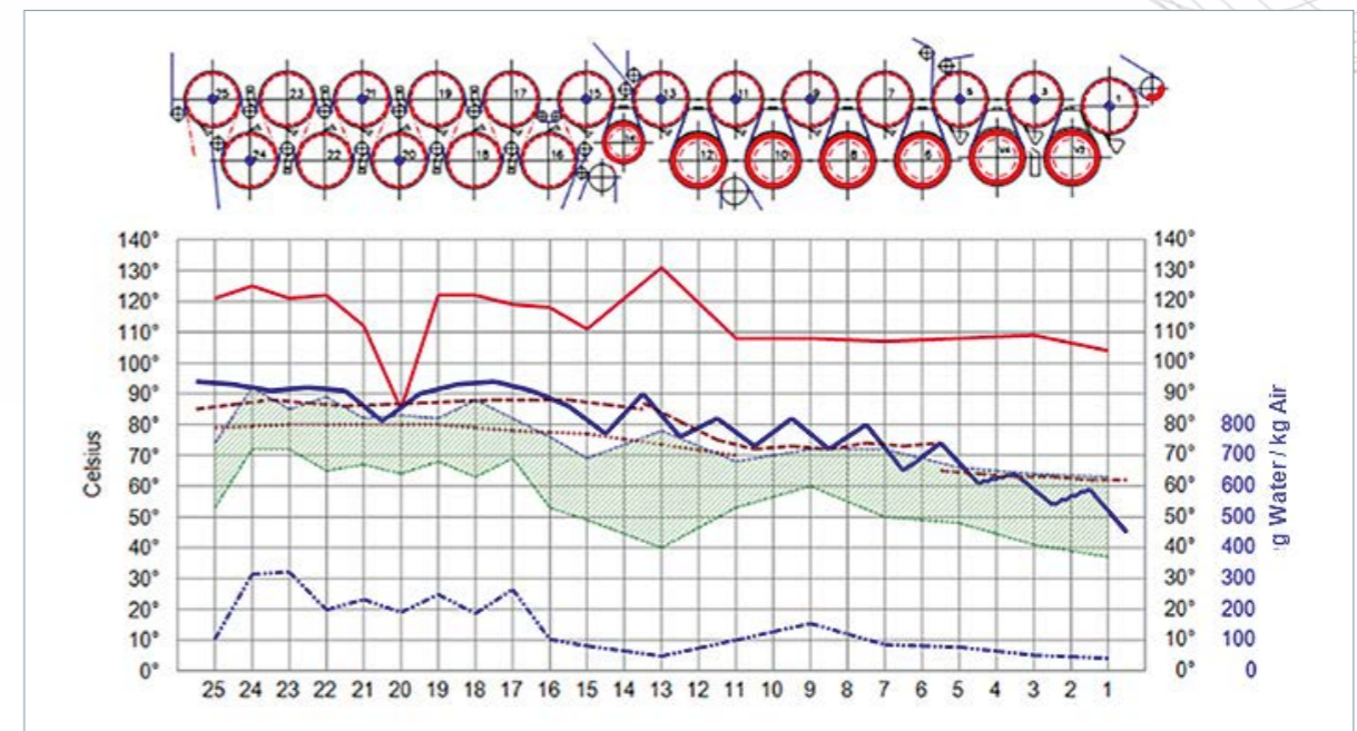
Fig. 6 : Diagramme de températures
