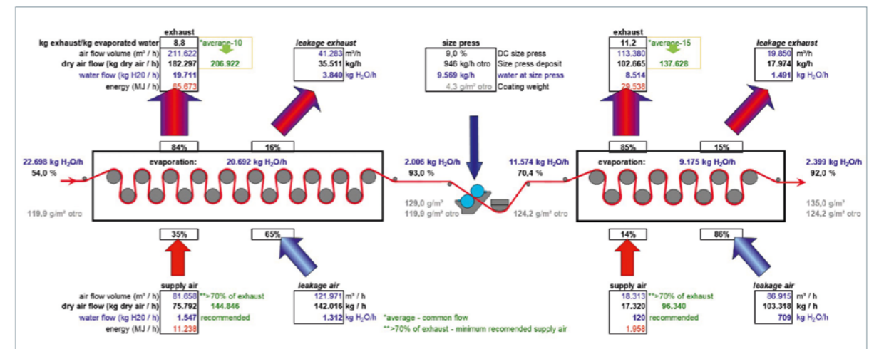
Fig. 7 : Bilan aéraulique
