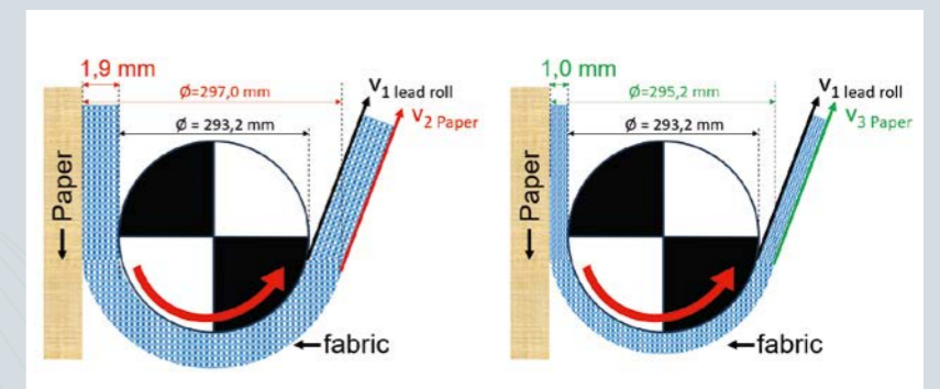
Fig. 12 : Influence de l'épaisseur toile sur la vitesse papier
