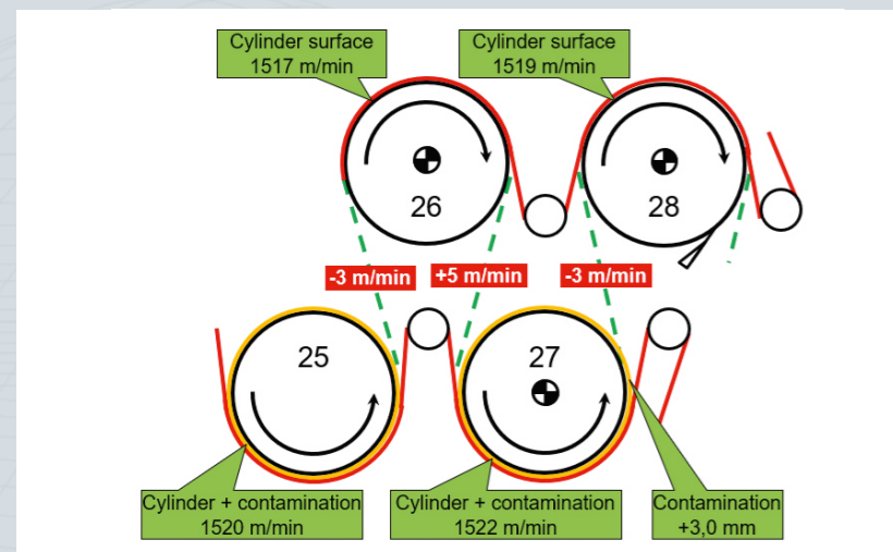
Fig. 9 : Vitesses périphériques mesurées
