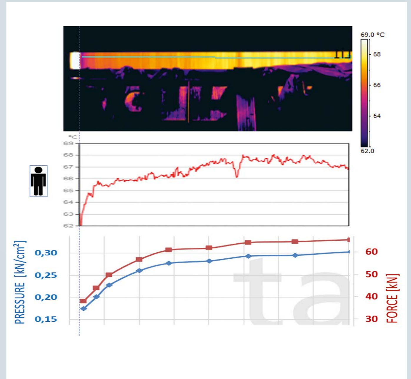
Fig. 15 : Feuille de papier sous le premier VacRoll; chute du profil de température sur le bord CC
