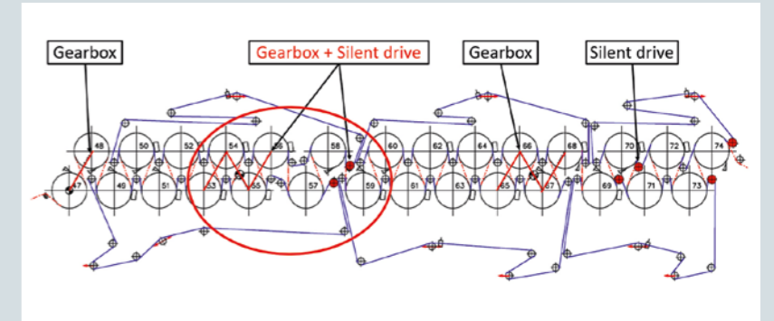
Fig. 10 : Schéma d'entraînement de la post-sécherie
