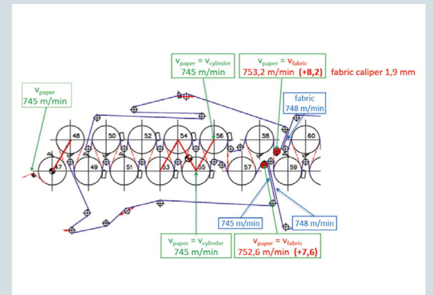
Fig. 11 : Modification des vitesses par le passage à des toiles plus fines
