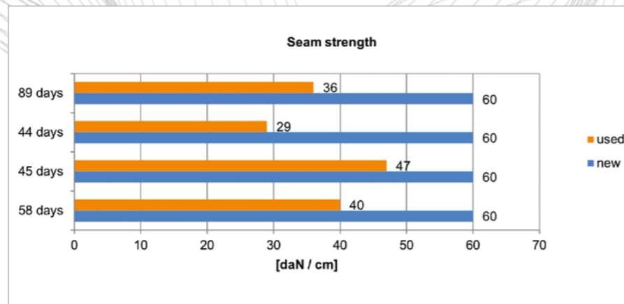
Fig. 3 : Historique de la résistance de la jonction
